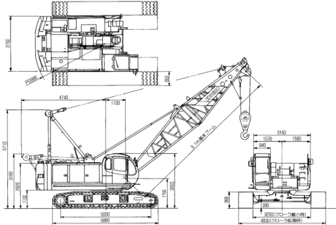
▶全体図(単位:mm)
